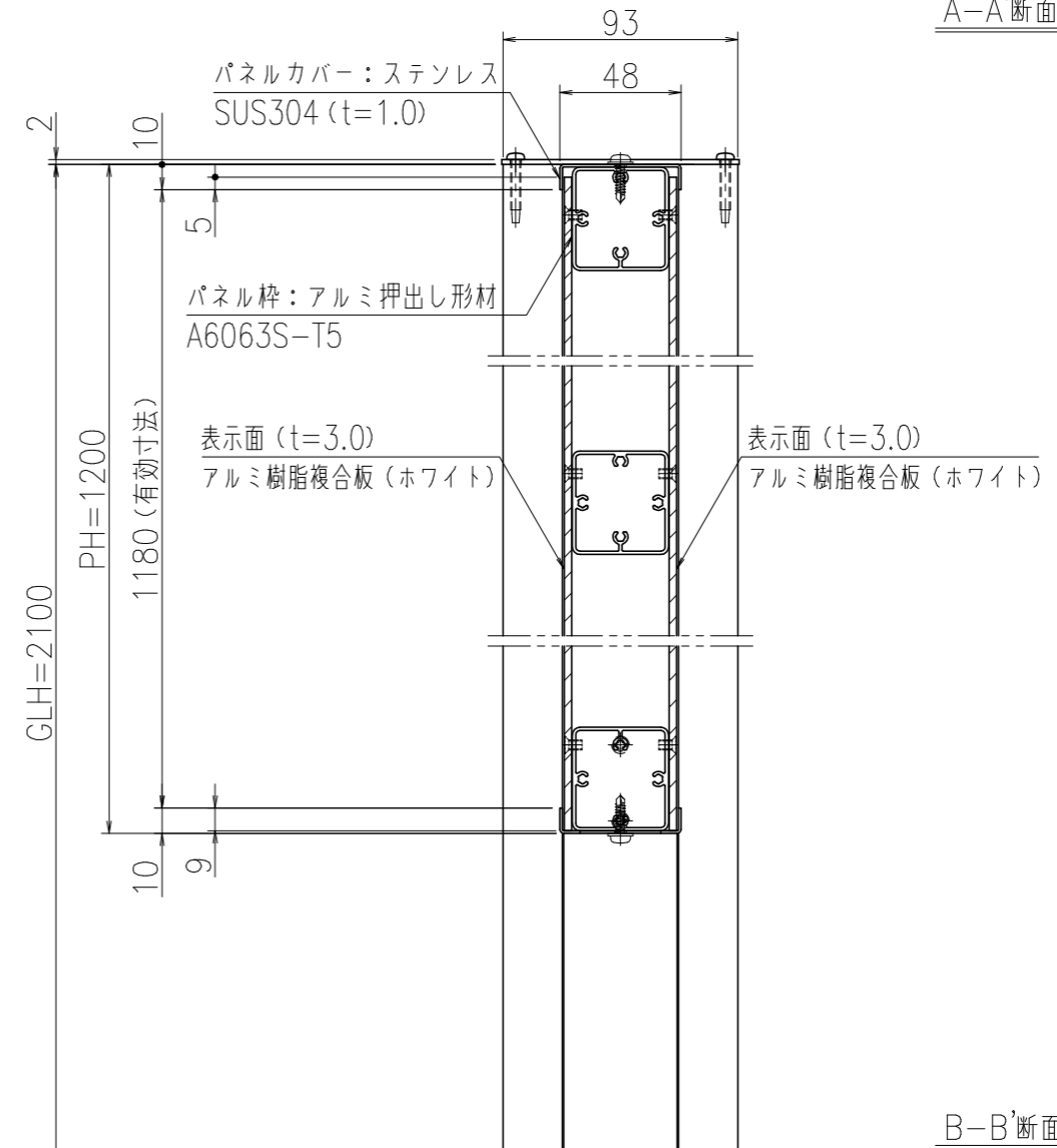
A-A'断面図 (S=1:3)
