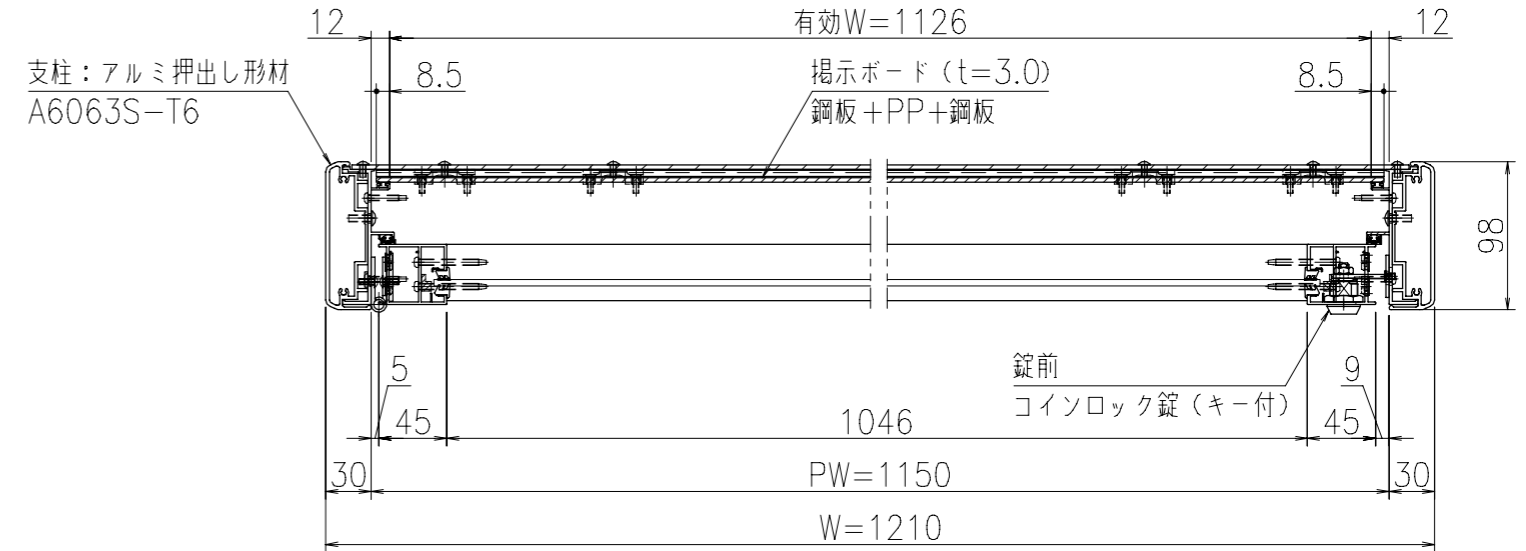
A-A'断面図 (S=1:5)
