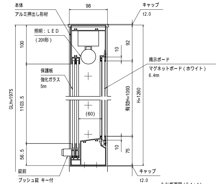
B-B' 断面図 (S=1:4)
