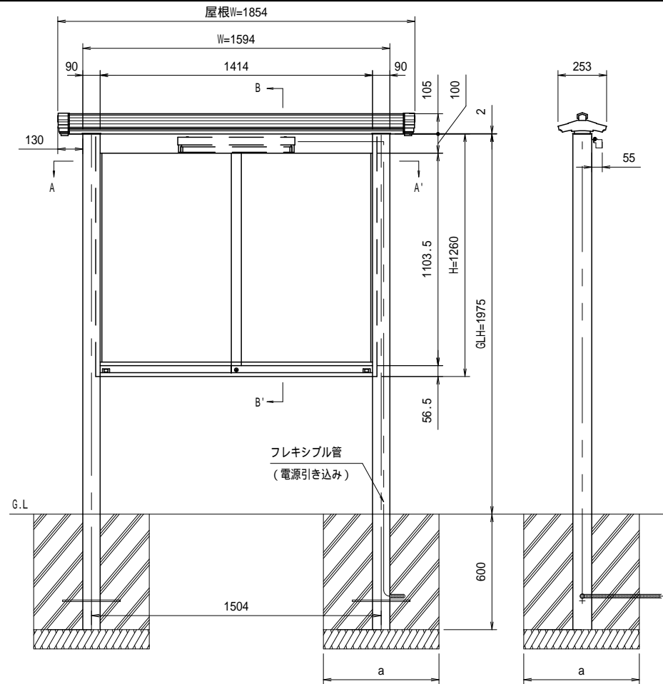
基礎寸法 a
