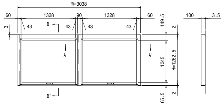
壁面取り付け穴寸法
