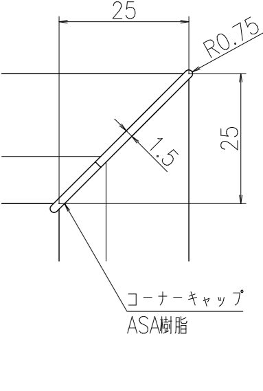
C部納まり図 (S=1:1)
