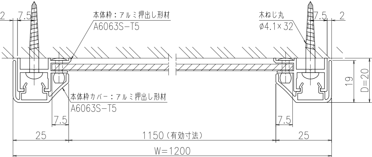
A-A断面図 (S=1:1)
