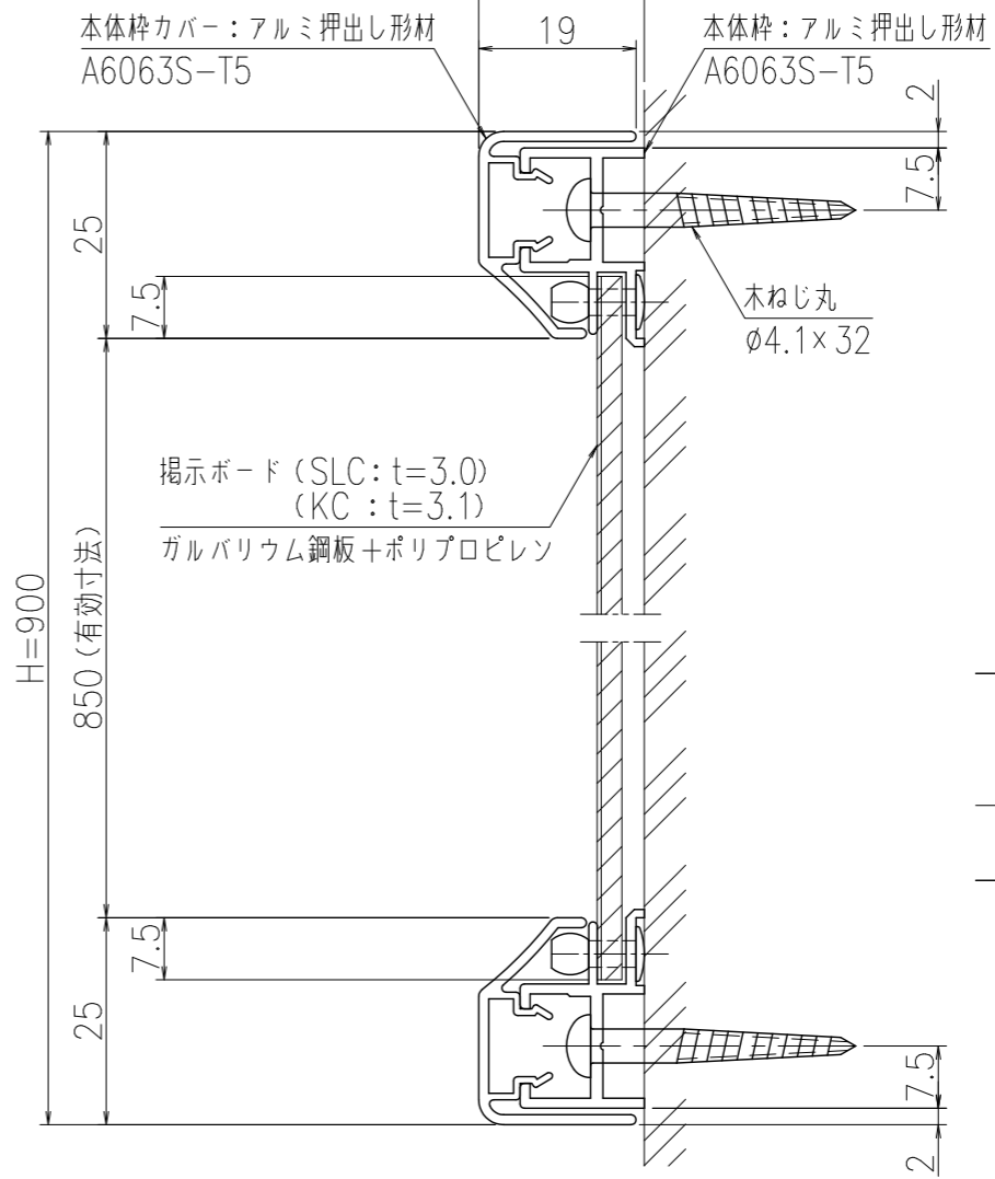
B-B'断面図 (S=1:1)
