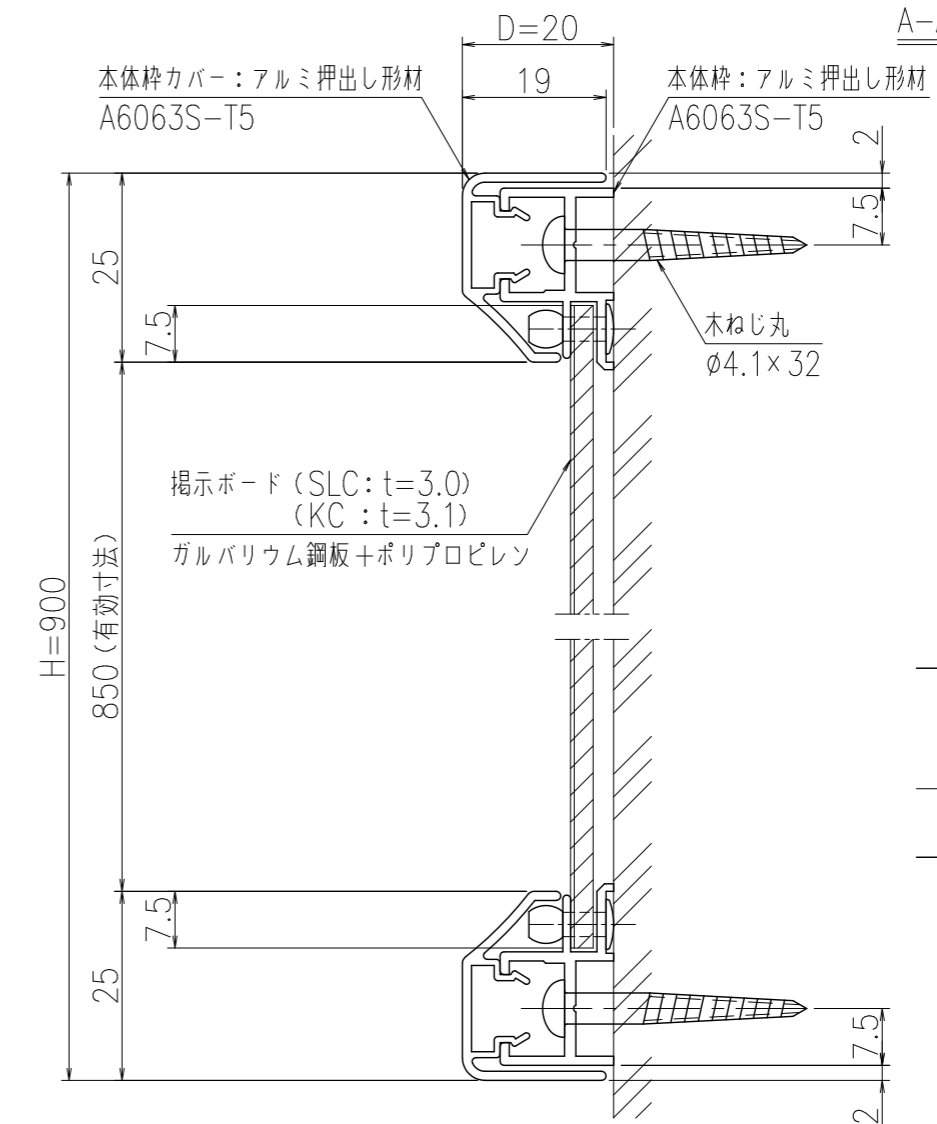
B-B'断面図 (S=1:1)
