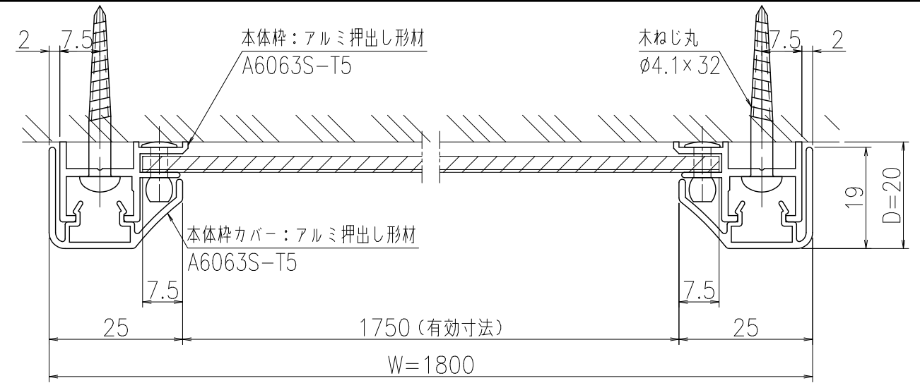
A-A断面図 (S=1:1)
