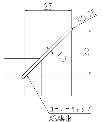
C部納まり図 (S=1:1)
