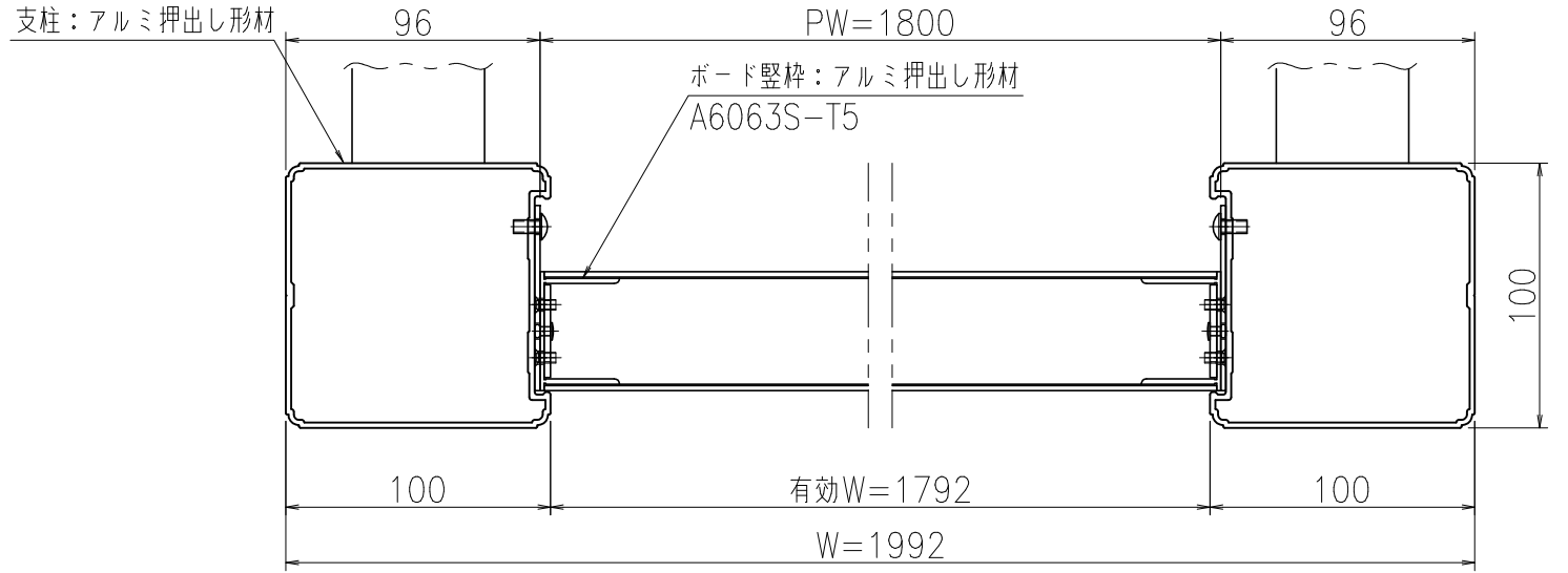
A-A'断面図 (S=1:3)
