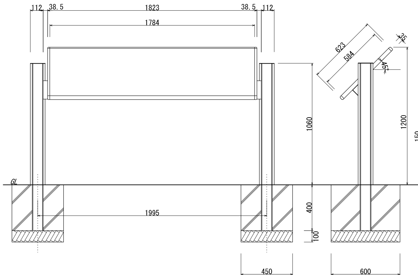
【正面図】
