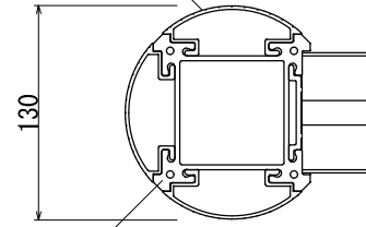
【丸支柱】
