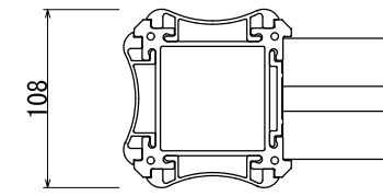
【X支柱】
