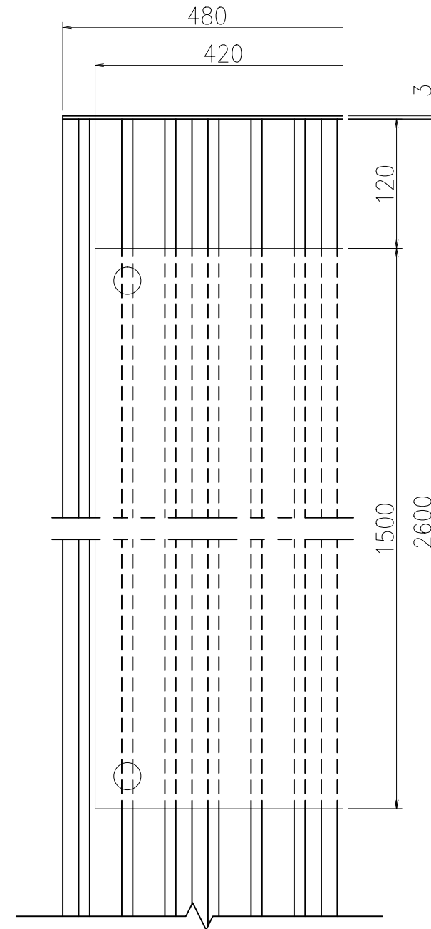
【正面図：タイプA】
