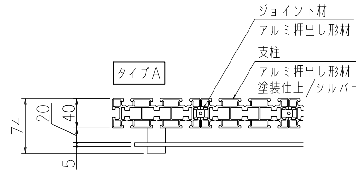
【平面図：タイプA】
