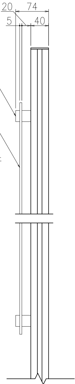
【側面図：タイプA】
