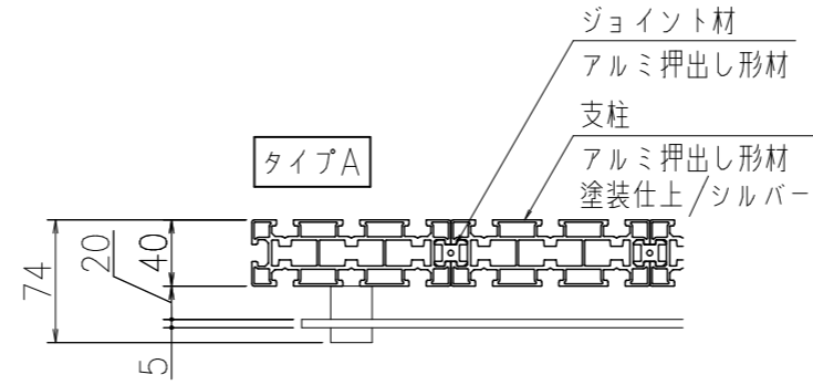
【平面図：タイプA】
