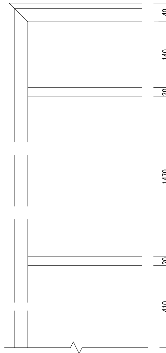
【正面図】
