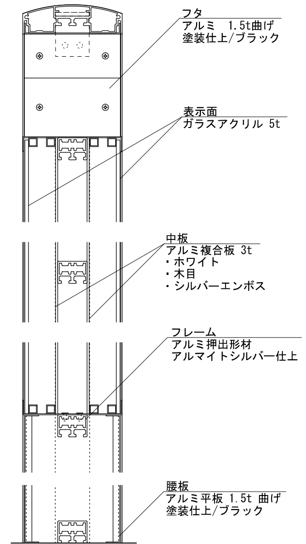
【側面図】
