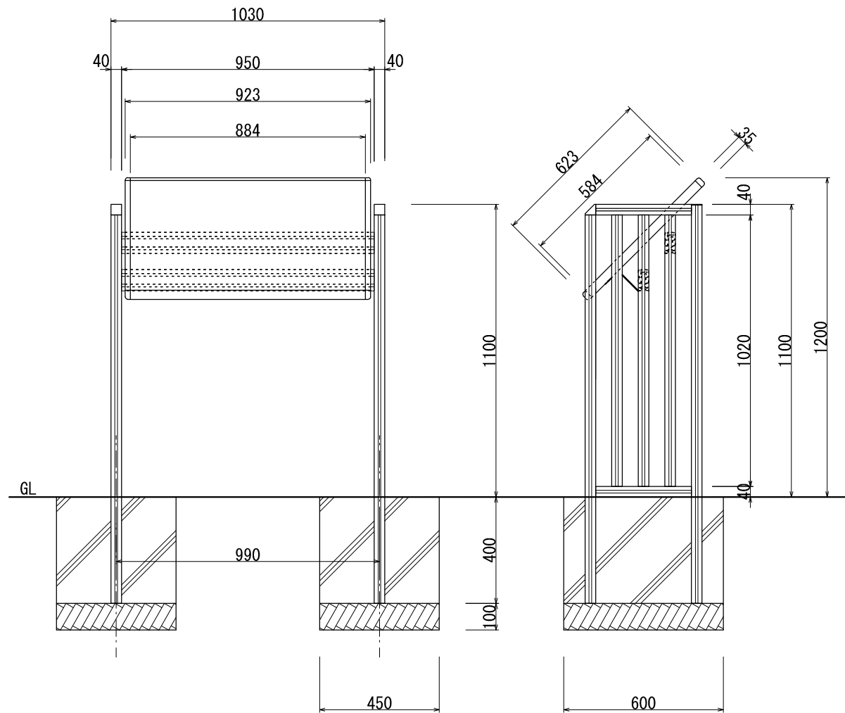
【正面図】
