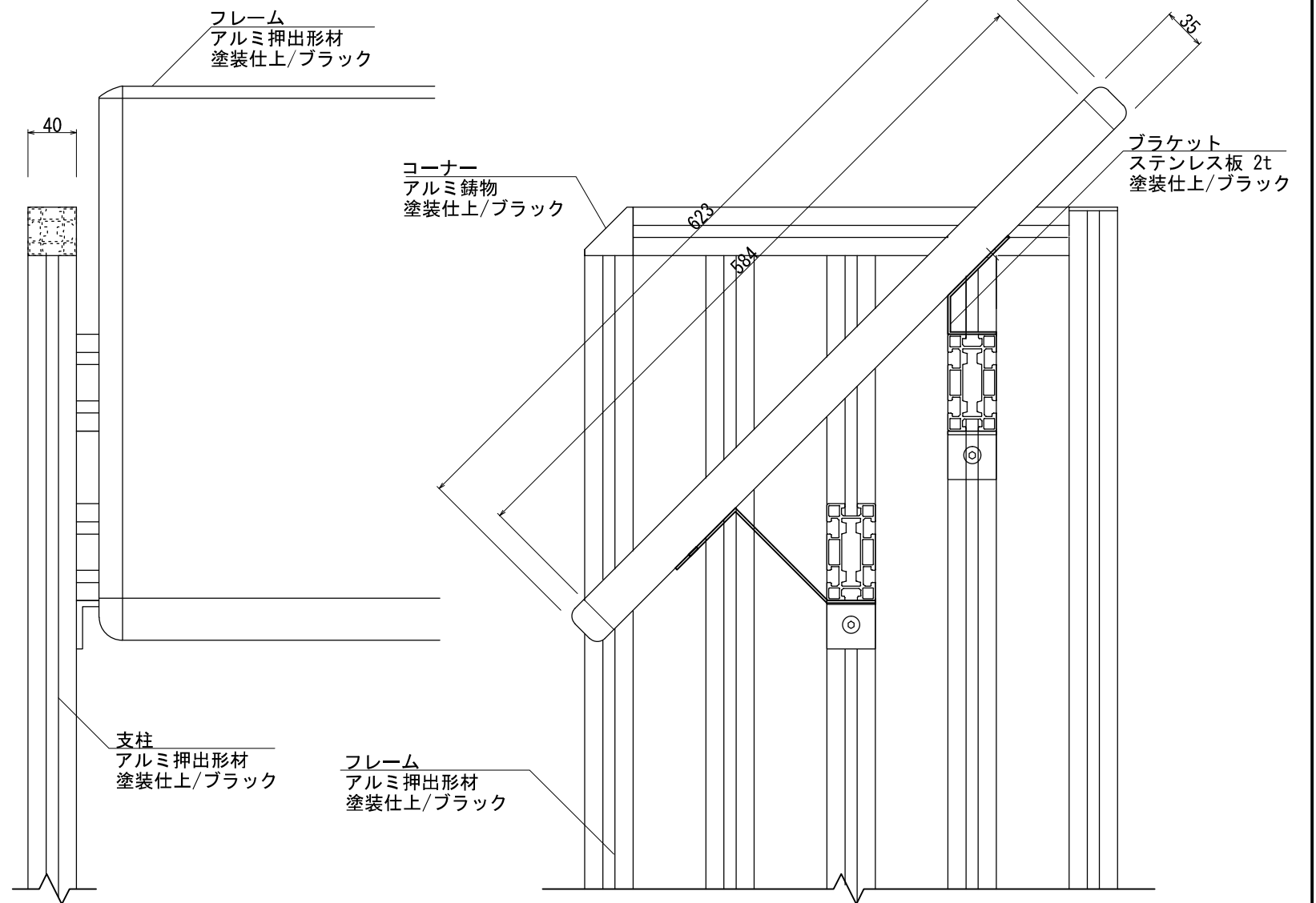
【正面図】
