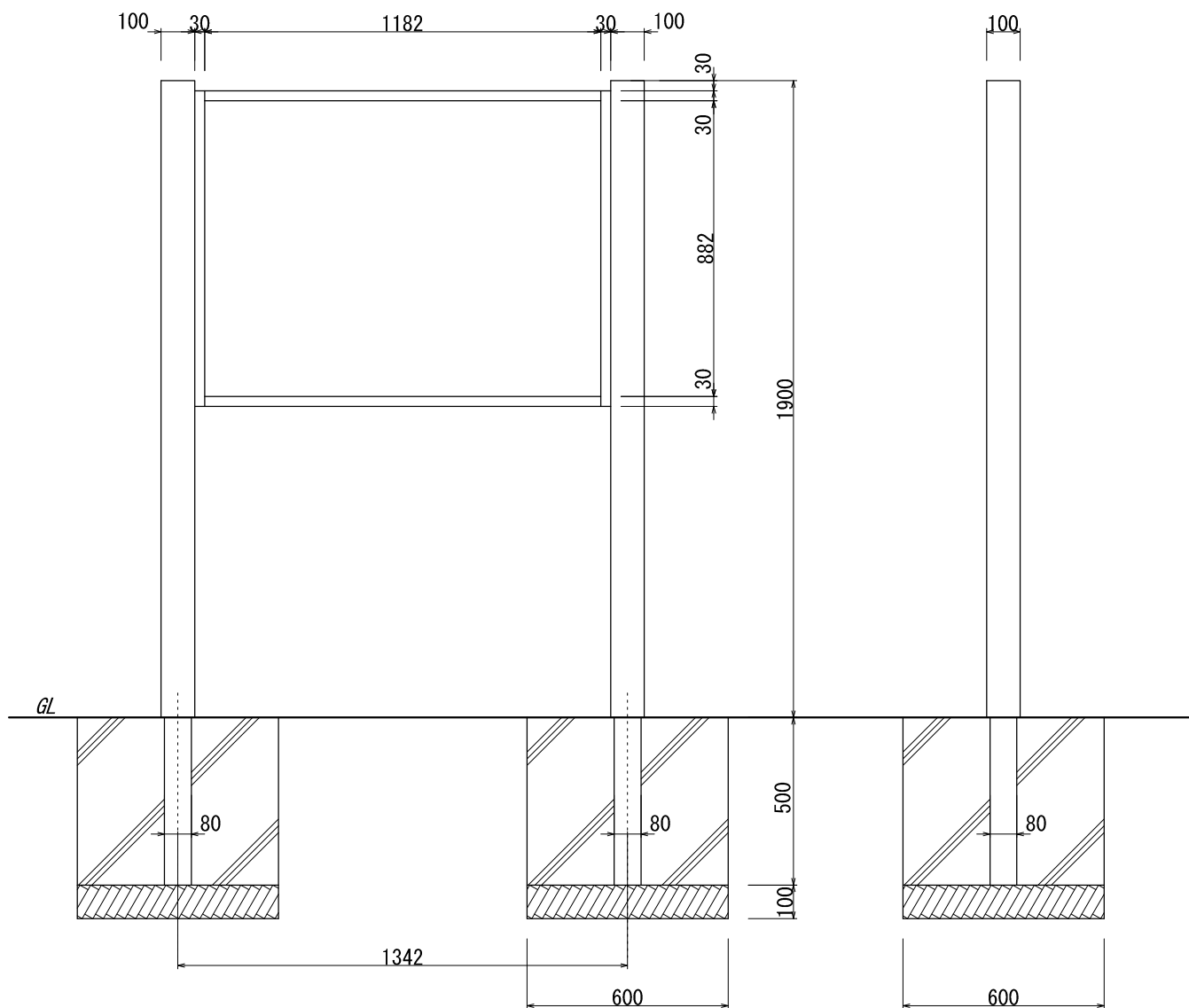
【正面図】
