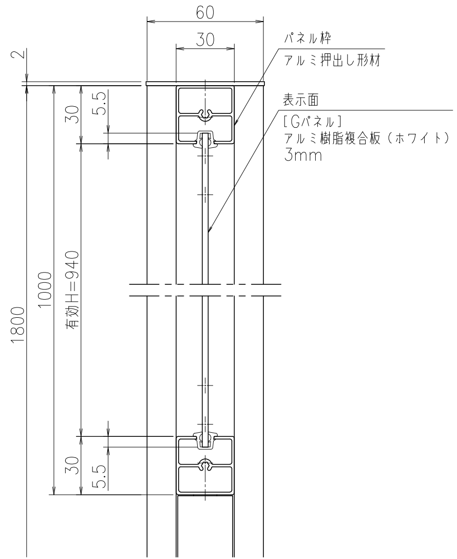
B-B'断面図 (S=1:2)
